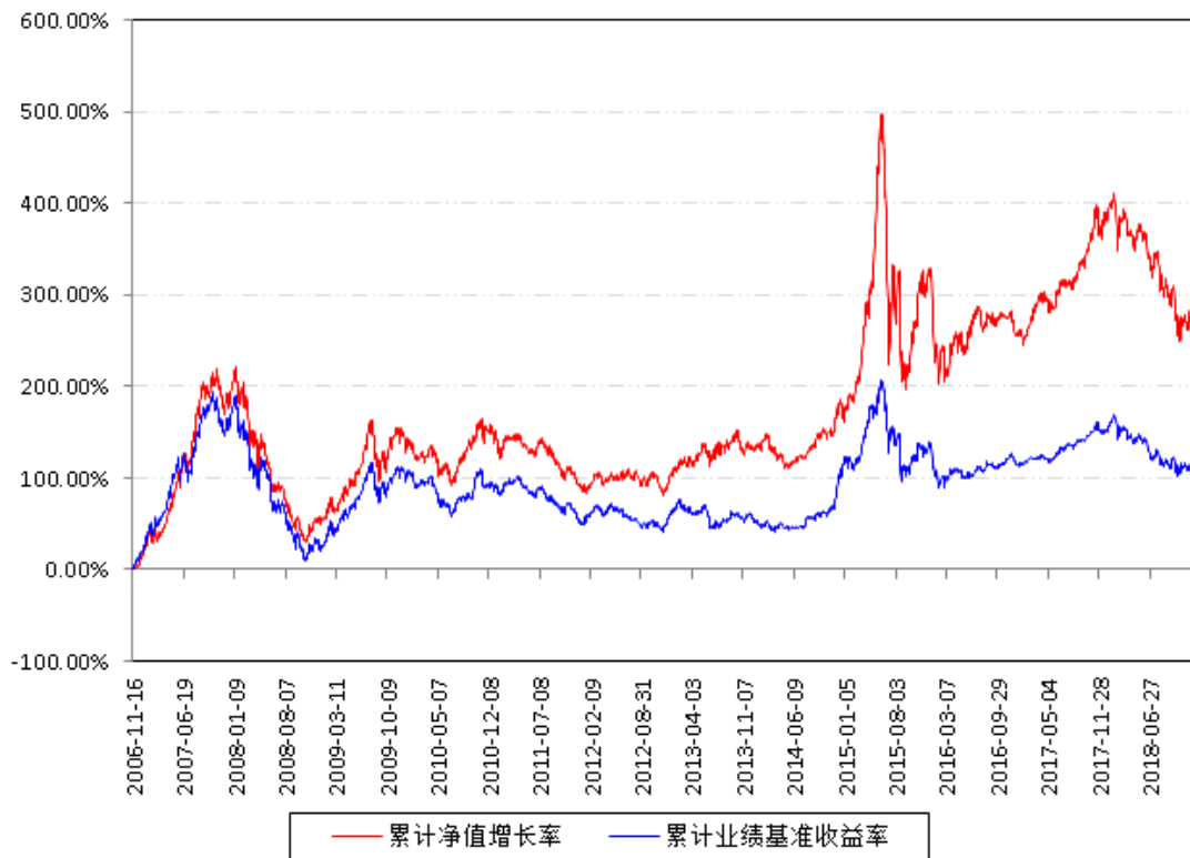
南方绩优A累计净值增长率与同期业绩比较基准收益率的历史走势对比图
